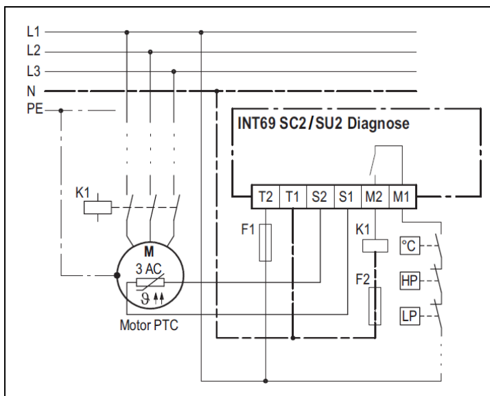
Рис. 19: Подключение модуля
