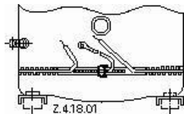
Рис. 15: Размещение нагревателя картера у компрессоров ZHI27K1P - ZHI46K1P
